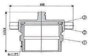
採水口啟動裝置：採水口ON/OFF+指示燈整組(cm)
