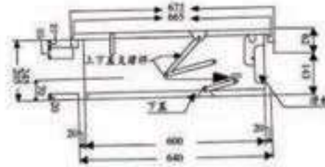
上視圖
